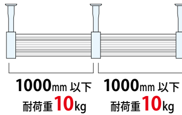
中間にブラケットを取付ける場合
