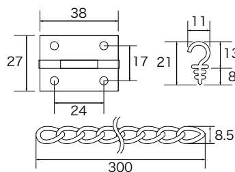
材 質：丁番 (鉄)38×27mm / 取付ビス (φ 2.7×8mm/ 鉄 / 皿タッピング) 開き角度調整チェーン (鉄) 洋灯フック (鉄) 全て塗装仕上
