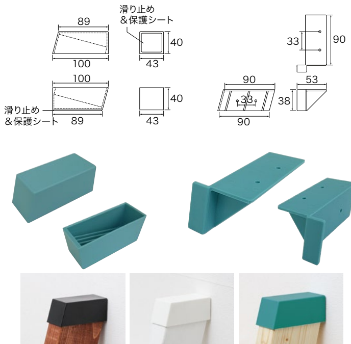
材 質：上部・下部・棚受パーツ (ABS 樹脂) ネジ (φ 3.5×16mm/ステンレス/トラスタッピング)
