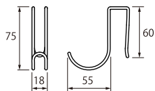
【1×4 専用フック】
